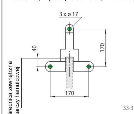
Mocowanie „H” prostopadle do tarczy hamulcowej
