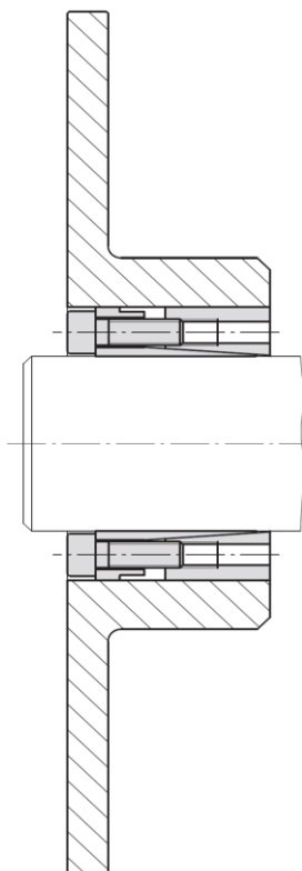
Pierścień rozprężno-zaciskowy RLK 130 z tarczą hamulcową typu B
