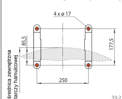
Mocowanie „V” równoległe do tarczy hamulcowej
