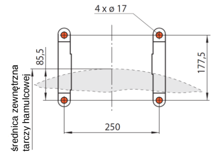
Mocowanie „V” równoległe do tarczy hamulcowej
