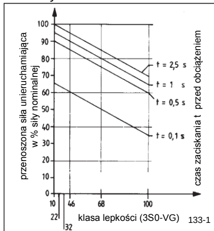
Zależność siły unieruchamiającej od lepkości oleju i czasu zaciskania przed obciążeniem (temperatura tłoczyska 20°C).
