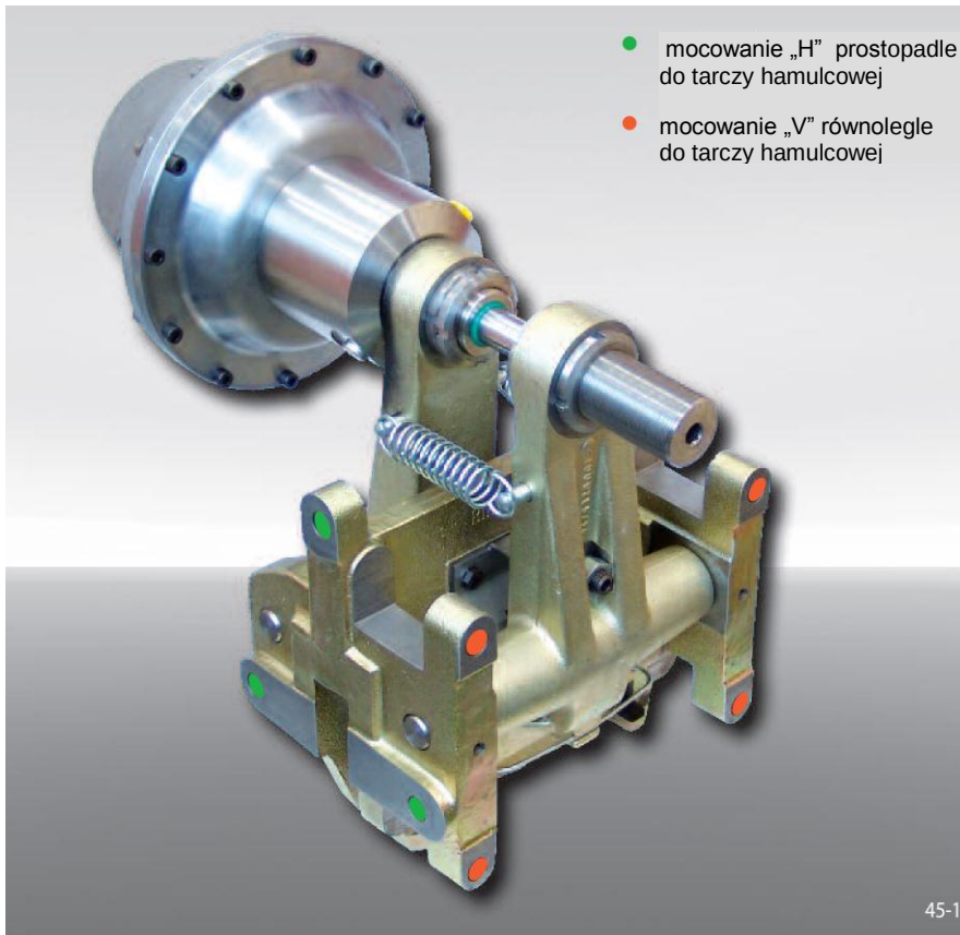
Mocowanie „V” równoległe do tarczy hamulcowej
