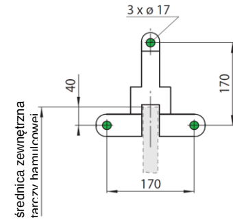
Mocowanie „H” prostopadle do tarczy hamulcowej
