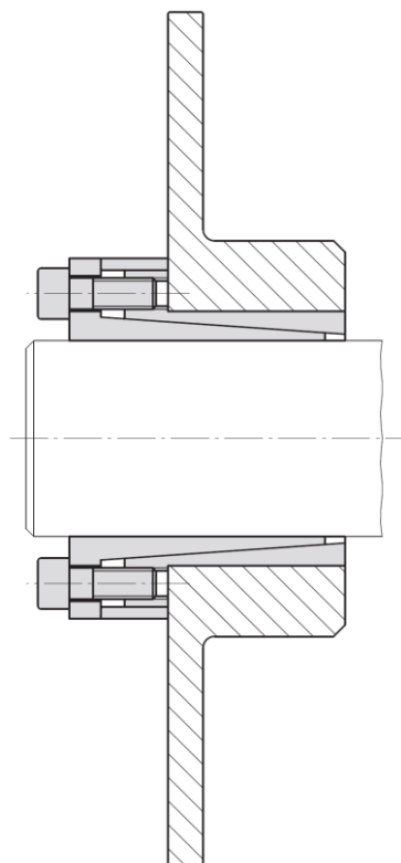
Pierścień rozprężno-zaciskowy RLK 110 z tarczą hamulcową typu B
