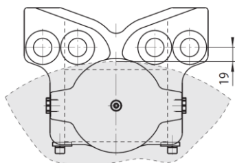
Montaż na tarczy hamulcowej 109-2
