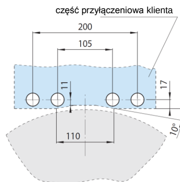
Wymiary części przyłącz. klienta 109-3
