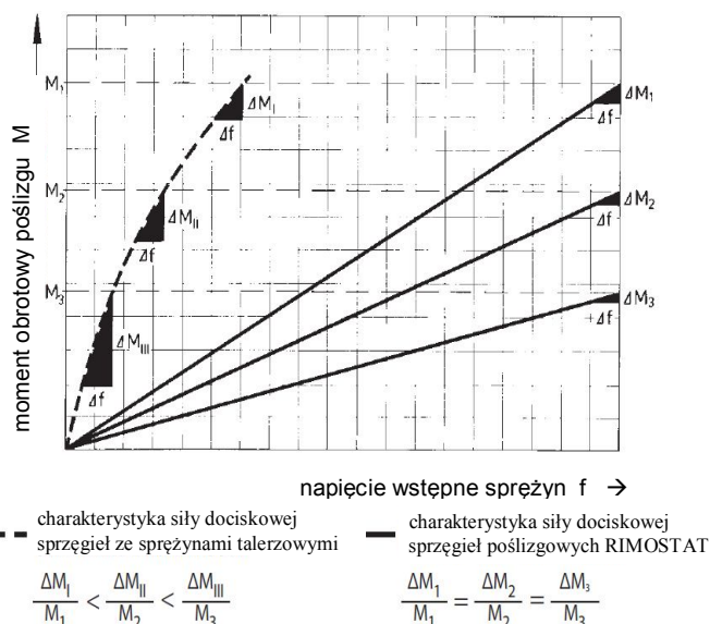
Mechanizm działania
