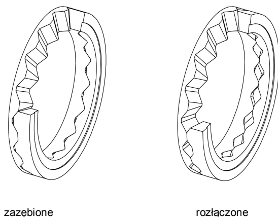
Mechanizm rozłączający
