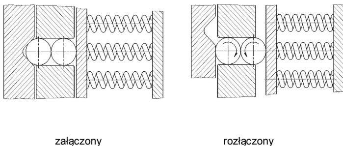
Zasada działania
