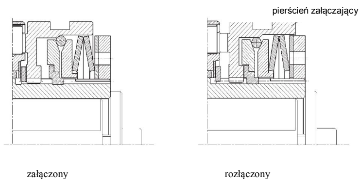
Mechanizm blokujący
