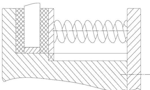
Mechanizm działania
