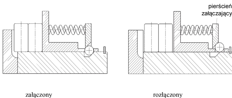
Mechanizm blokujący
