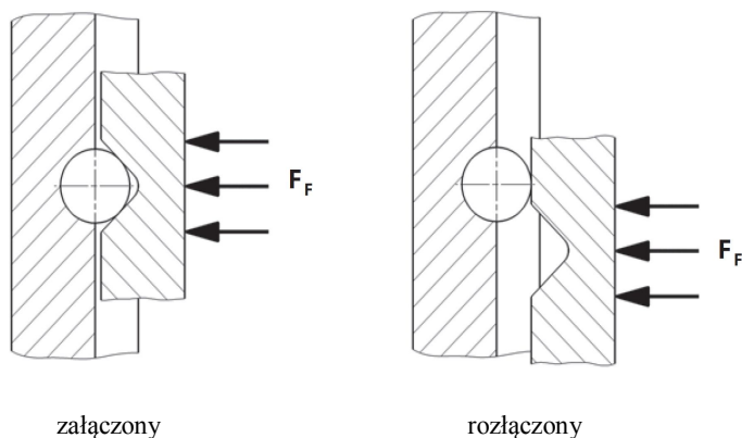
Zasada działania
