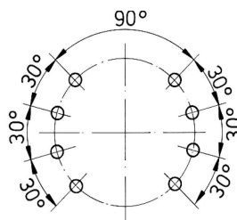
Układ otworów 3
