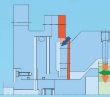
Uchwyt zaciskowy z membraną głęboką - strona 42
