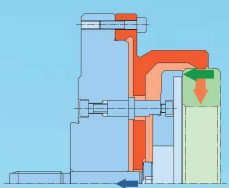
Uchwyt zaciskowy z membraną segment. - strona 42
