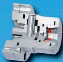
Uchwyt kołnierzyowy z zestawem tarcz zacisk. - strona 12 - 19
