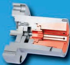
Uchwyt kołnierzyowy z tuleją stożkową - strona 20 - 25
