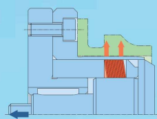
Trzpień do mocowania z tuleją rozprężną - strona 85
