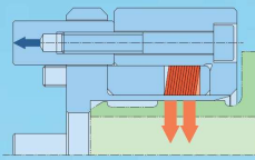
Uchwyt zaciskowy z tuleją rozprężną - strona 43
