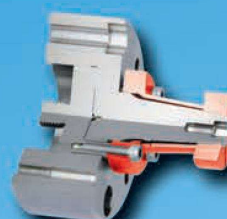
Trzpień kołnierzyowy z oprawką stożkową - strona 62 - 67
