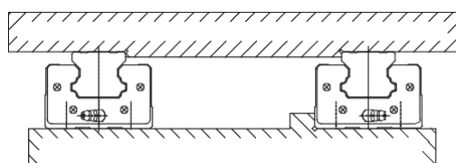
Dwie szyny profilowe z wózkami zamontowanymi na stałe
