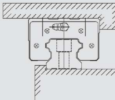
Szyna profilowa przy krawędzi oporowej
